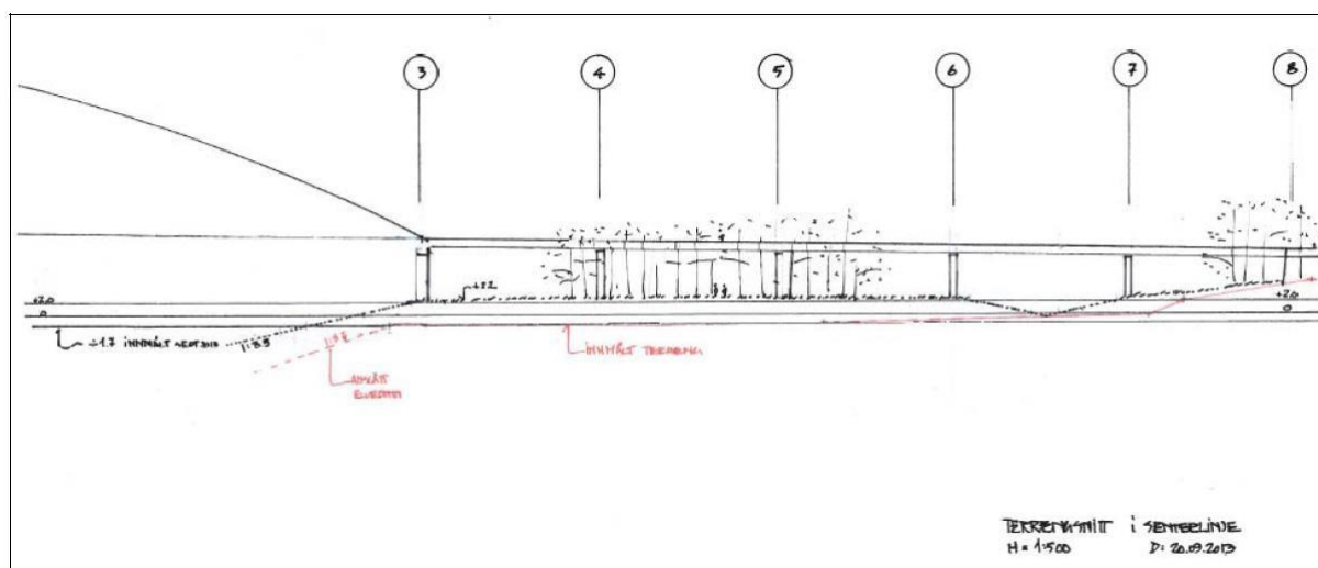
Figur 16 - Skisse/lengdesnitt for fylling under viadukt
