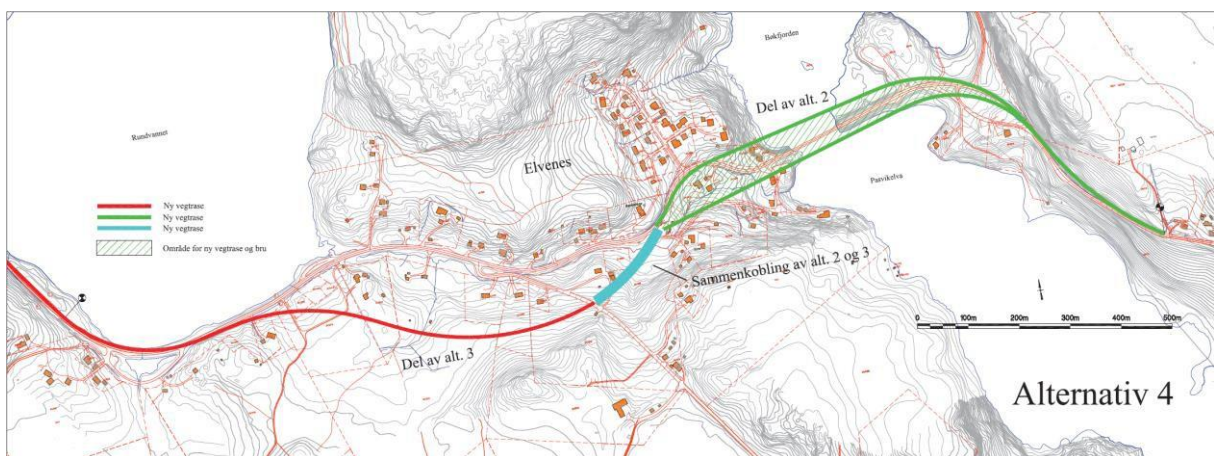
Figur 4 - Alternativ 4: Kombinasjon av alternativ 2 og 3
