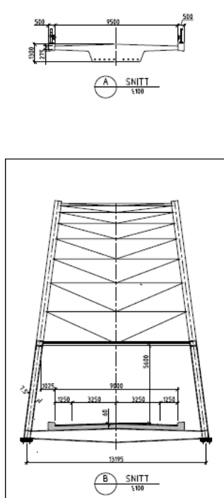
Figur 11 - Snittegninger - ny bru over Bøkfjorden
