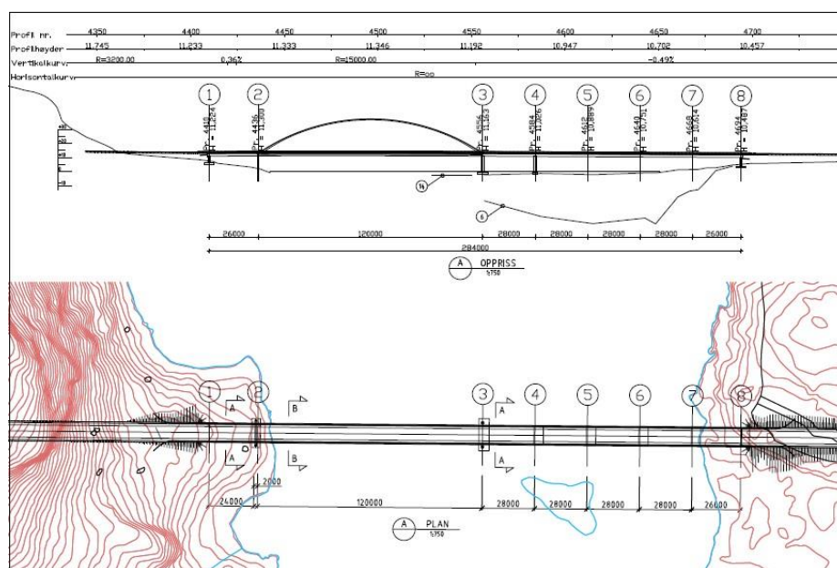
Figur 10 - Oppriss og plan for ny bru over Bøkfjorden
